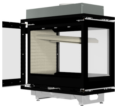
Verwijder de eerste rookgeleidingsplaat
