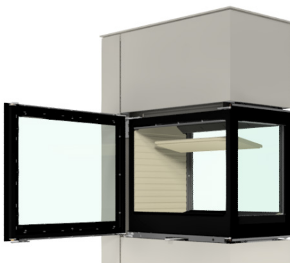
Verwijder de bovenste rookgeleidingsplaat
